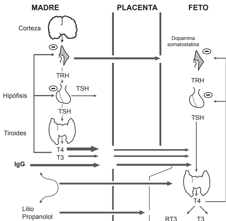
Fig. 7.2. Eje hipófisis-tiroideo durante la gestación y la unidad funcional materno-feto-placentario. Durante el embarazo, existen tres ejes funcionales tiroideos: el de la gestante, la placenta y del feto. Trabajan paralelamente y pueden interactuar entre ellos
